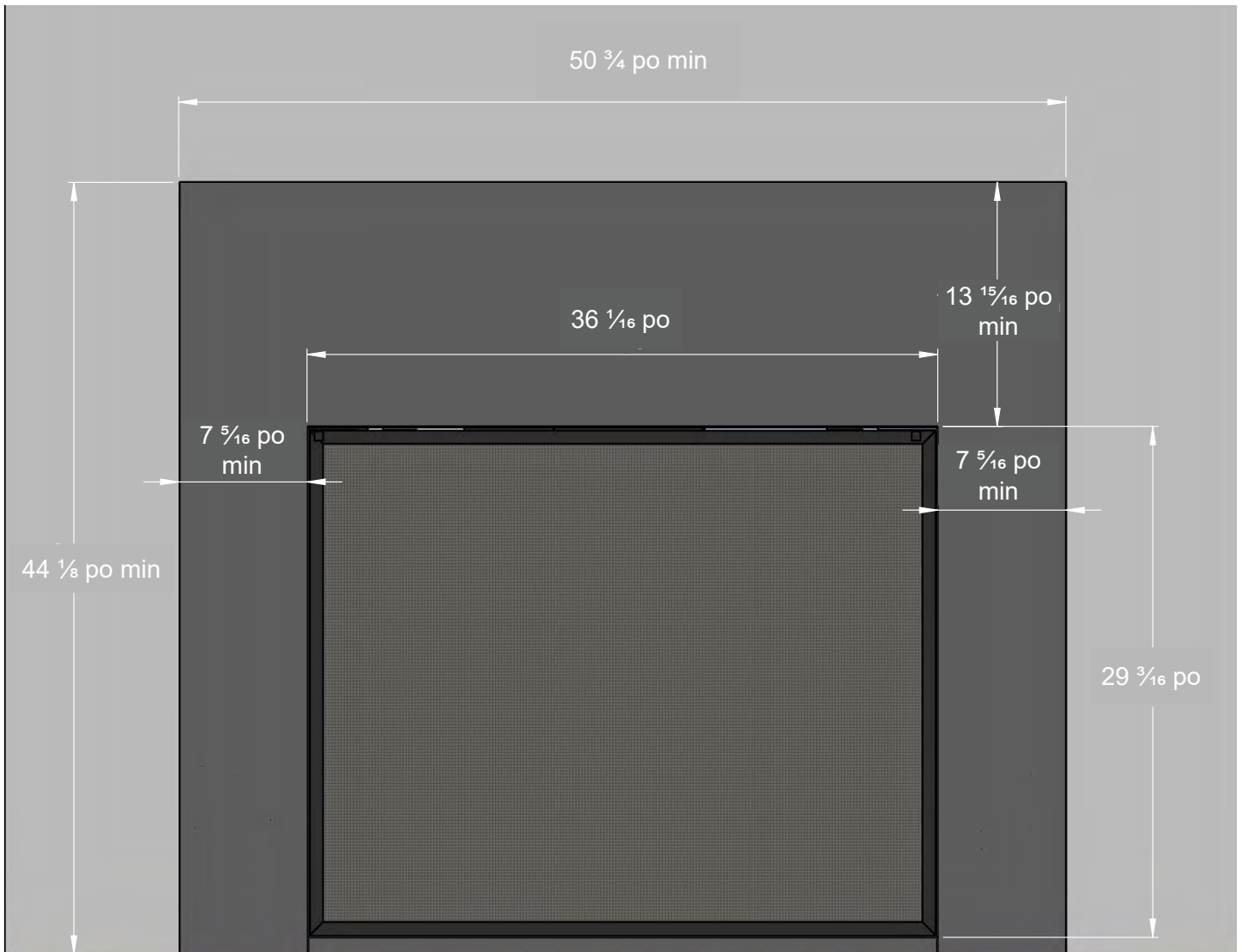
Figure 12.4.07: Dimensions du matériau incombustible sur la face du foyer
