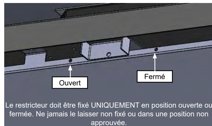
Figure 10.2.03: Restricteur non sécurisé.
