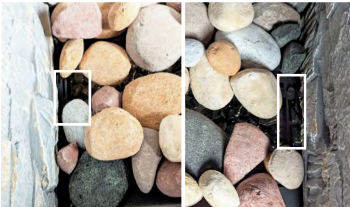
Figure 2.3.03: Ouvertures d'air secondaire
